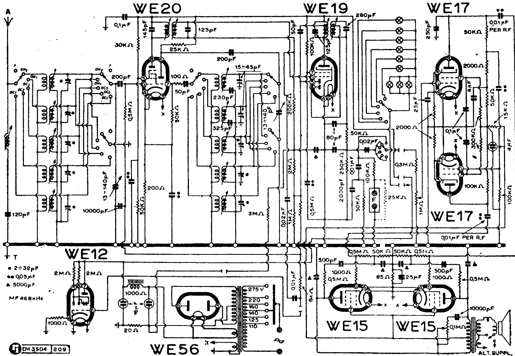
COMP. RADIORIC. TELEFUNKEN - MODD. « T 8 » « T 8 RF »
